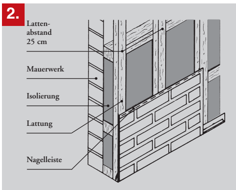
Aufbau mit Isolierung
