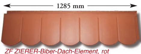
Dachsanierung mit ZF ZIERER-Leichtdachelementen
