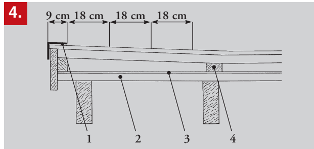
1 Ortgang angehoben, 2 Schalung, 3 Dachpappe, 4 Konterlatte
