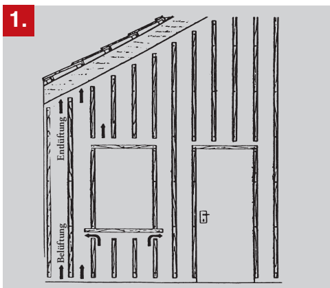
Be- und Entlüftung beachten!
