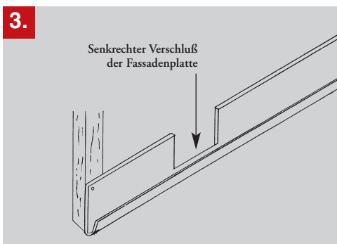
Starterleiste, Länge 3200 mm
