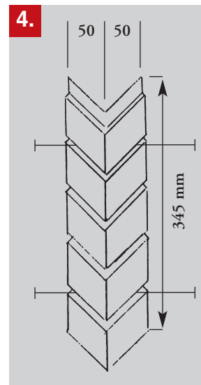
ZF ZIERER-Original-Ecken Befestigung mit Fugennägeln
