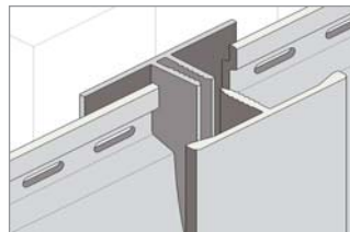
H-Profil (2-teilig)
