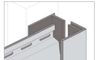
U-Profil (2-teilig)
