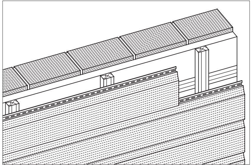
vinylPlus Fassadenprofil
